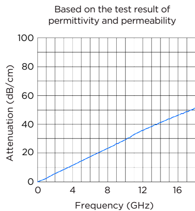
Attenuation
